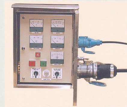
遠隔操作盤
